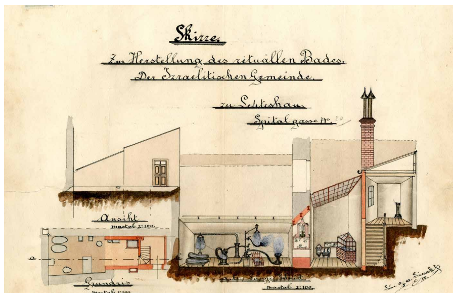
Projekt židovských rituálnych kúpeľov na Špitálskej ulici č. 20 v Levoči z roku 1903 (Zdroj: Spišský archív v Levoči)
